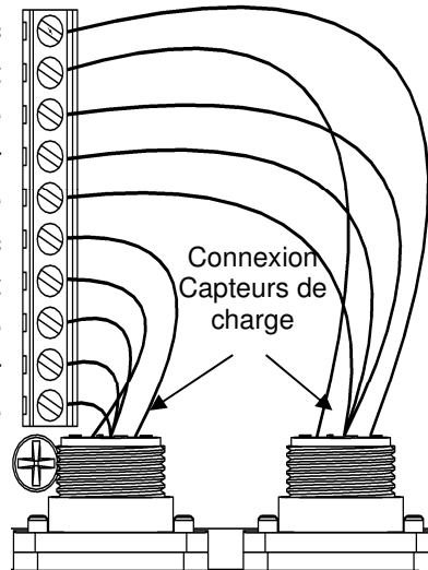
Diagramme Connexion des conducteurs
